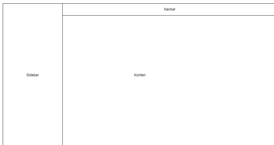
Gambar 3.12 Rancangan Antarmuka
